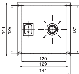
Steuergerät STG1/ control unit STG1 Gewicht/ weight: 0.3 kg
