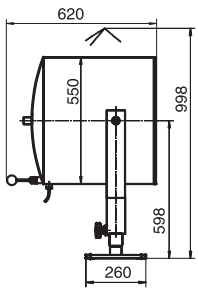
NHS550A Gewicht/ weight: 23.3 kg
