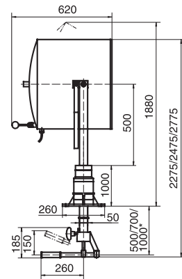
NHS550D Gewicht/ weight: 32.0 kg
