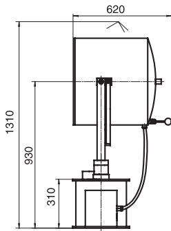
NHS550F Gewicht/ weight: 48.0 kg
